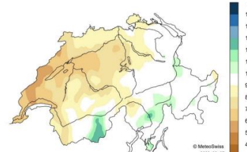
Abb 4: Räumliche Verteilung der Niederschlagssumme im Sommer 2023 (Juni bis August) dargestellt in % der Norm 1991-2020.
