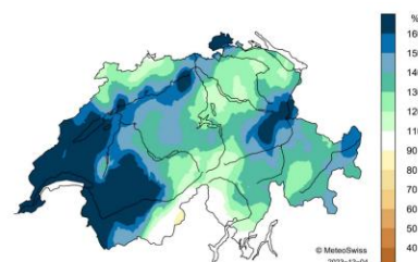
Abb 6: Räumliche Verteilung der Niederschlagssumme im Herbst 2023 (September bis November) dargestellt in % der Norm 1991-2020.
