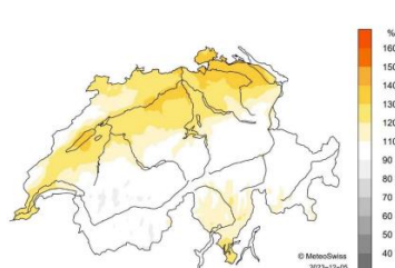
Abb 5: Räumliche Verteilung der Sonnenscheindauer im Herbst 2023 (September bis November), dargestellt in in % der Norm 1991-2020.
